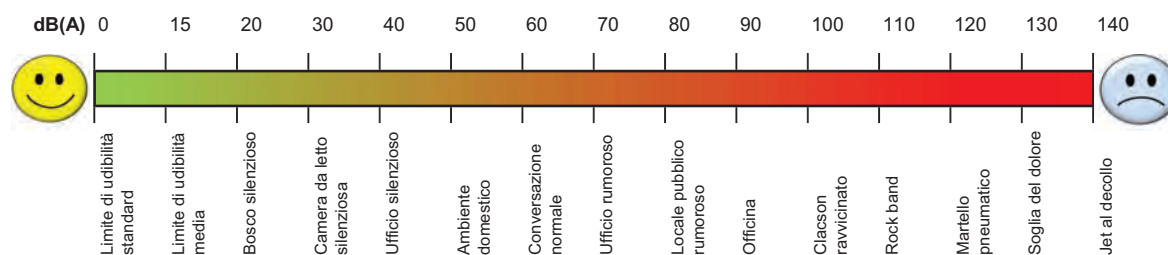
FIGURA 2 - SCALA DEL RUMORE IN RELAZIONE ALLA SENSIBILITÀ UDITIVA
